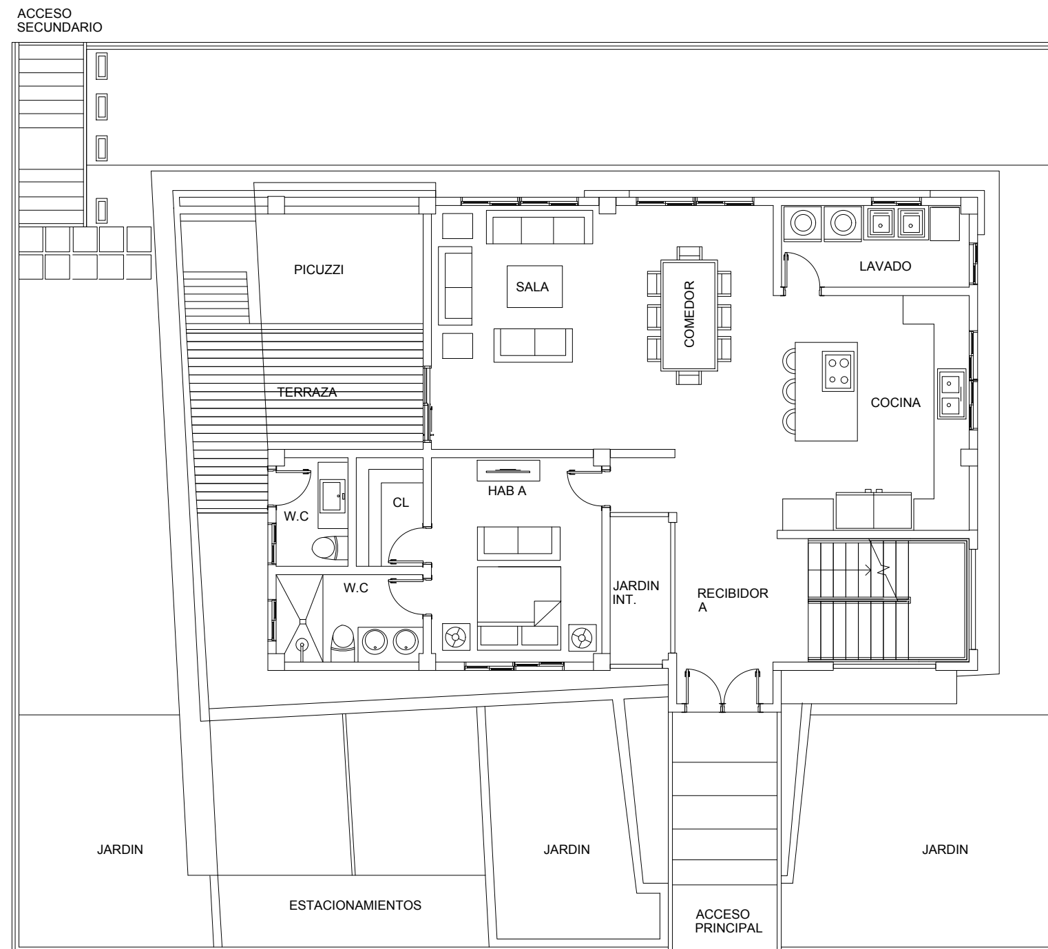
PLANTA AMUEBLADA NIVEL 1
